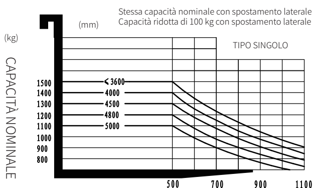
CPD15TVL POSIZIONE DEL CENTRO DI CARICO (mm)
