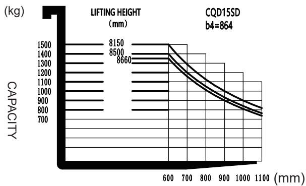
CENTRO DE CARGA(mm)
