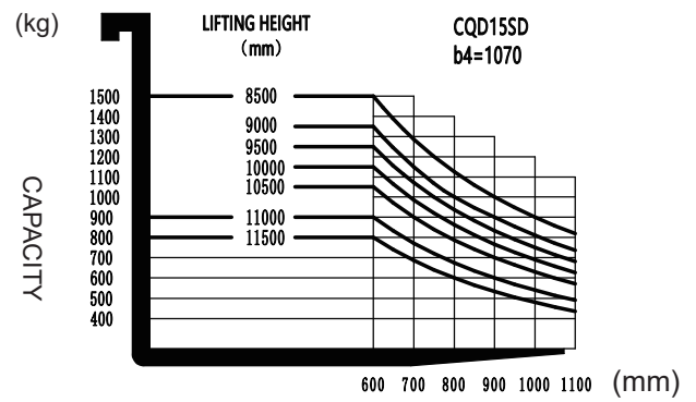
CENTRO DE CARGA(mm)
