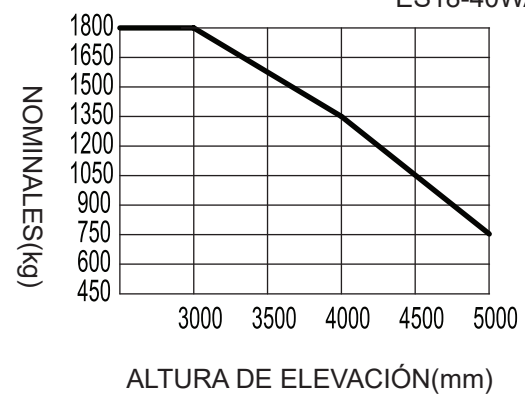
GRÁFICO DE CAPACIDADES NOMINALES ES18-40WA
